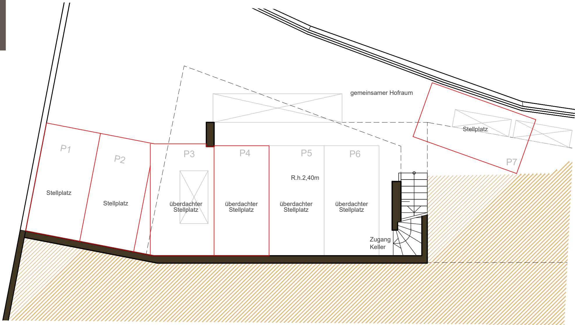
Kellergeschoss
