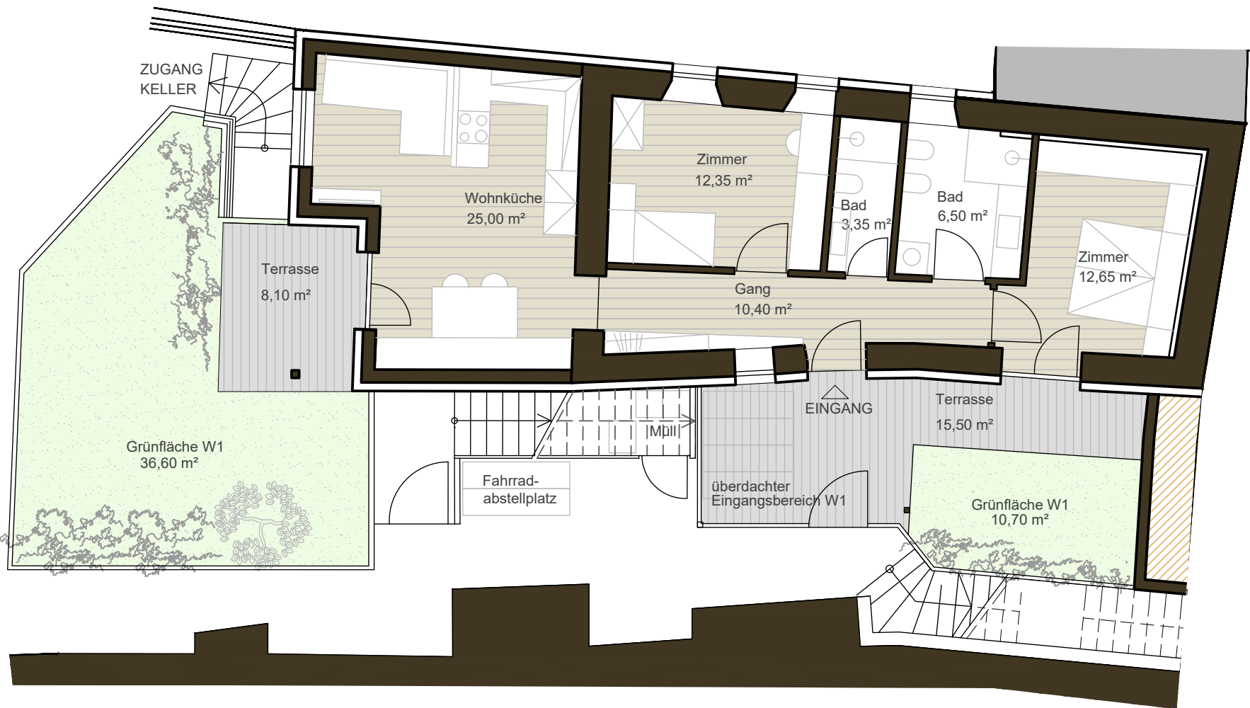
Erdgeschoss
